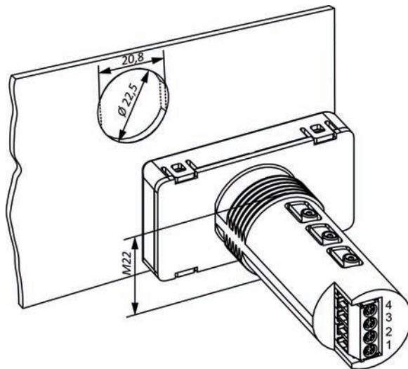
Рисунок А.2 – Установка прибора в отверстие сложной
