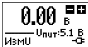
Рисунок 4.3 – Экран прибора в режиме измерения напряжения
