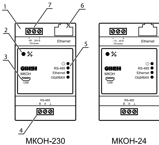
Рисунок 2 – Общий вид прибора
