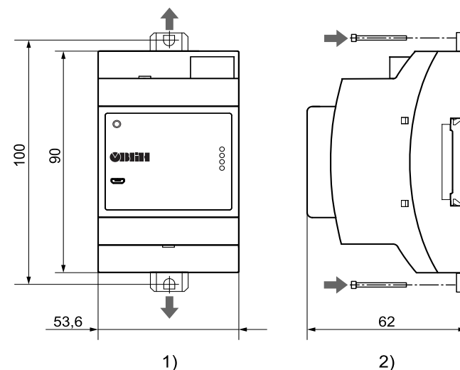
Рисунок 1 – Габаритные и установочные размеры
