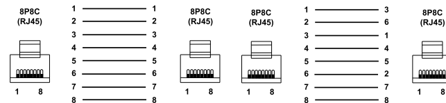
Рисунок 3 – Схема прямого кабеля для соединения прибора по сети Ethernet
