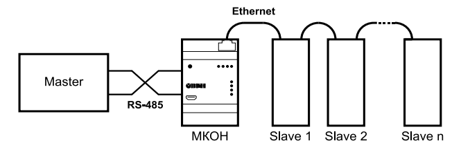
Рисунок 6 – Использование шлюза с Мастером сети в интерфейсе RS-485
