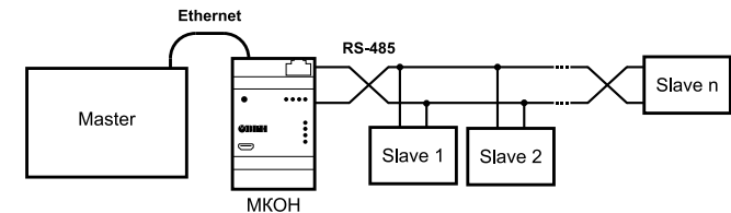
Рисунок 5 – Использование шлюза с Мастером сети в интерфейсе Ethernet
