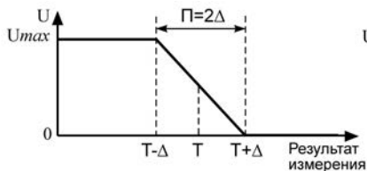
а) обратно-пропорциональное регулирование
