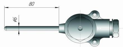
Рисунок 1 – Термопреобразователь Т.п/п – Кл3–1
