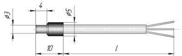
Рисунок 1 – Термопреобразователи сопротивления ТСПг и ТСМг в конструктивном исполнении К0
