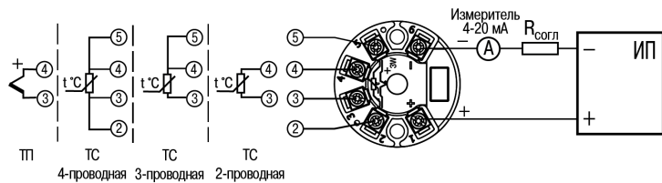
Рисунок 6.3 – Подключение прибора
