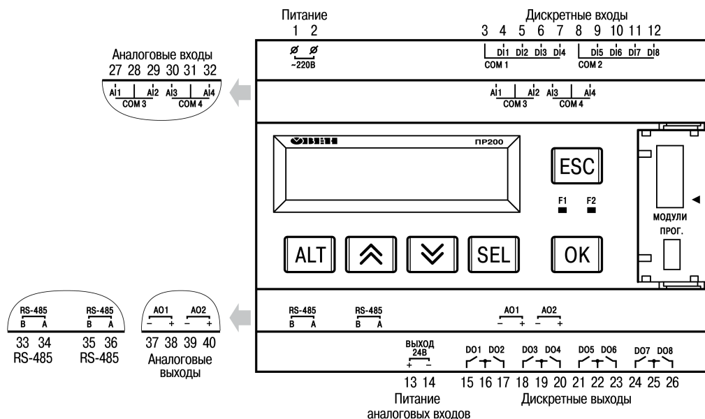
Рисунок 5.8 – Расположение контактов и элементов индикации в приборе ПР200-220.2(22).Х
