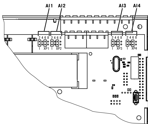
Рисунок 7.4 – Схема расположения перемычек
