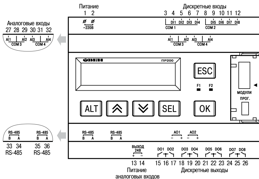
Рисунок 5.9 – Расположение контактов и элементов индикации в приборе ПР200-220.3(23).Х
