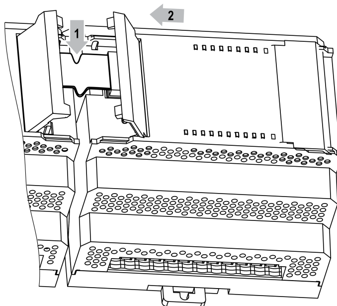
Рисунок 5.29 – Укладка шлейфа в углубление
