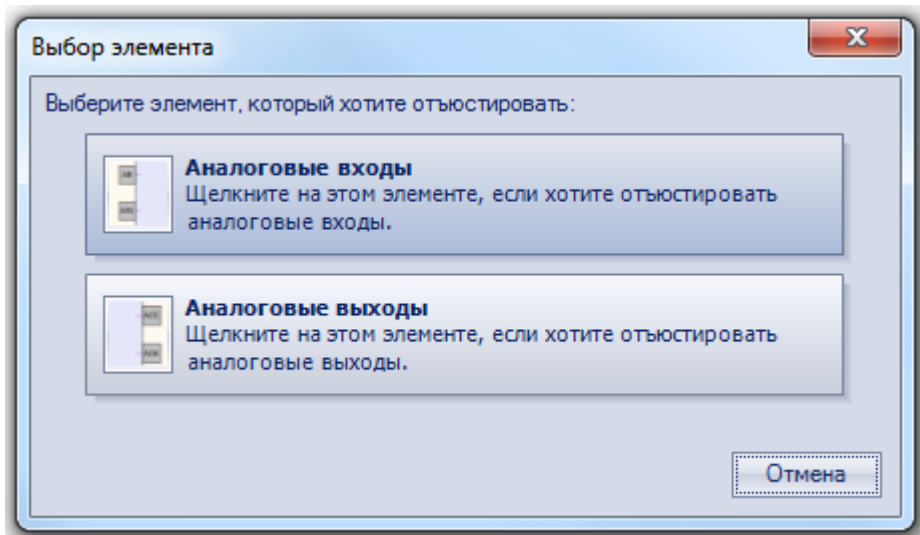
Рисунок 8.5 – Выбор элемента
