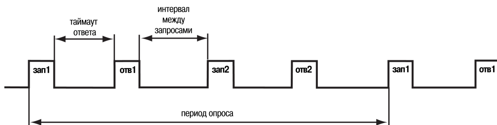
Рисунок 7.13 – Порядок запросов
