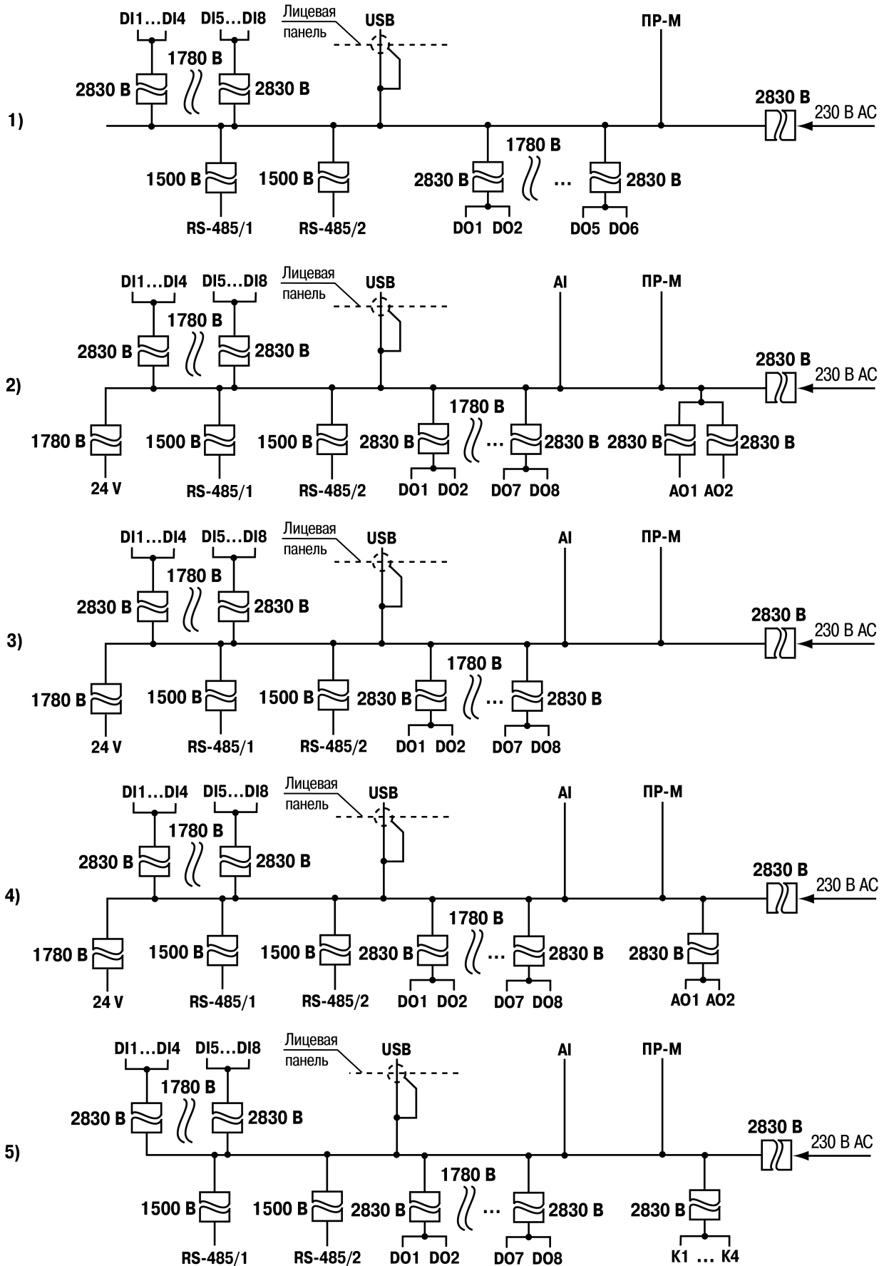
Рисунок 5.2 – Схема гальванической развязки: 1) PR200-220.1(21).X.X, 2) PR200-220.2(22).X.X, 3) PR200-220.3(23).X.X, 4) PR200-220.4(24).X.X, 5) PR200-220.5(25).X.X
