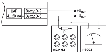
Рисунок 8.7 – Подключение ВУ1 типа И ( R_H=500 Ом)
