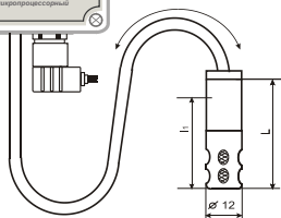
Настенное исполнение – Н2
