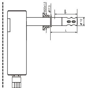
Настенное исполнение – Н2
